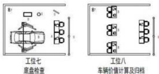
图 5 机动车鉴定与评估作业模块场地布置图（以现场为准，部分工位合并）
