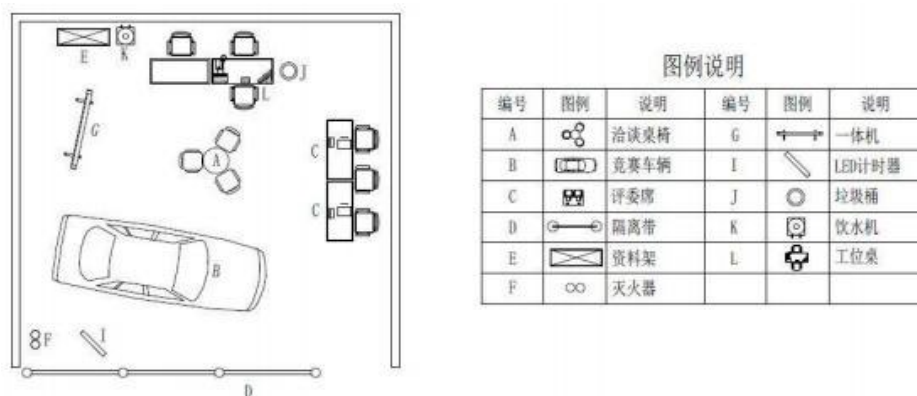
图 4方案展示、在线说车与展厅体验式销售场地布置图
