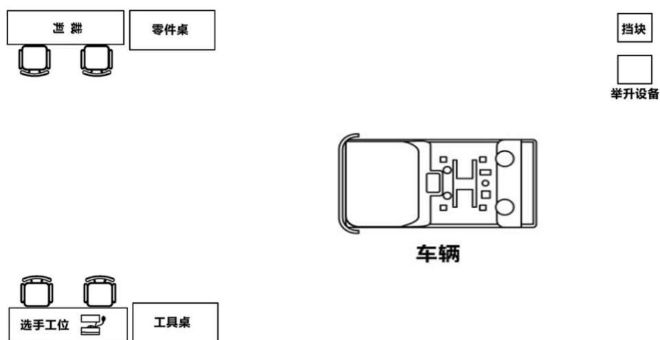
图 1 模块一工位布置图（以实际场地为准）
