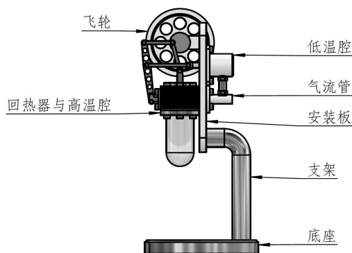
图 1-4 斯特林发动机基本组成
