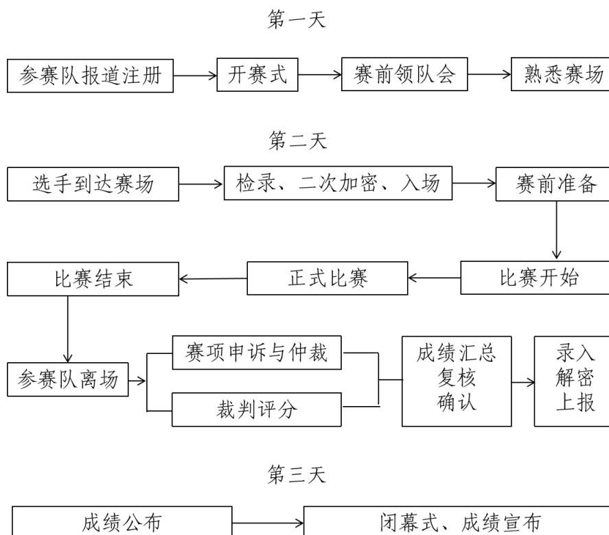
图1 竞赛流程图
