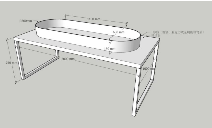
图 2 容器空间示意图
